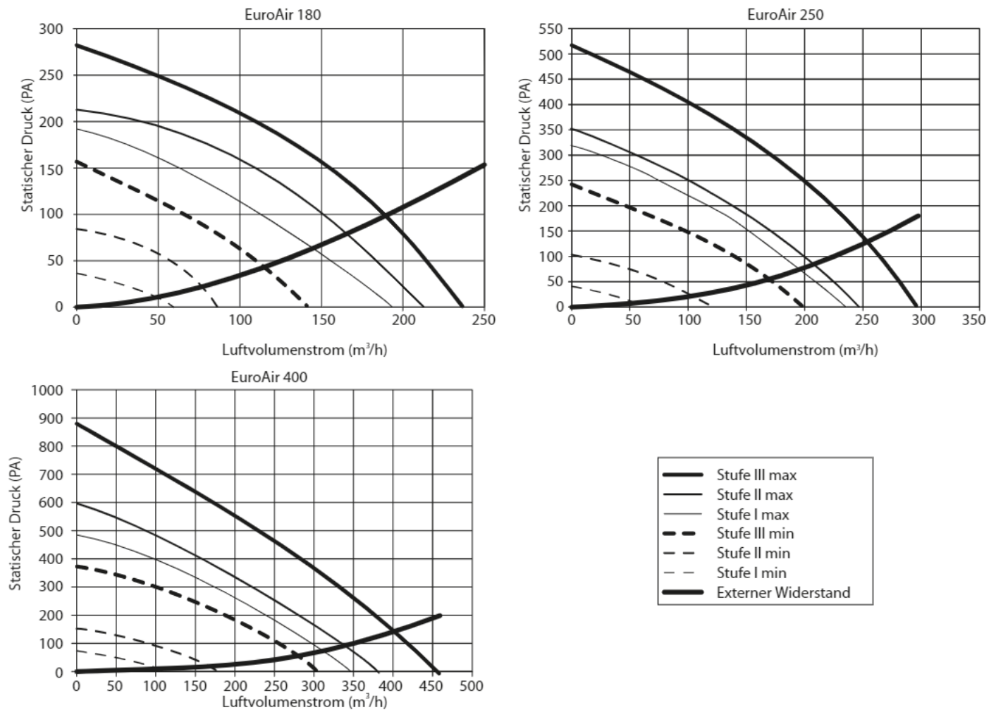
Darstellung Steuerspannung-Luftvolumenstrom externe Pressung des EuroAir 180, 250 und 400
